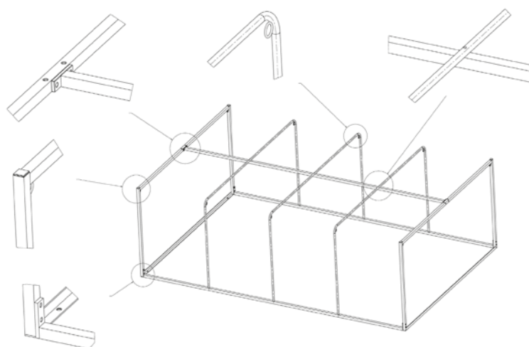
Windschutzbox freistehend für Bodenbeete
